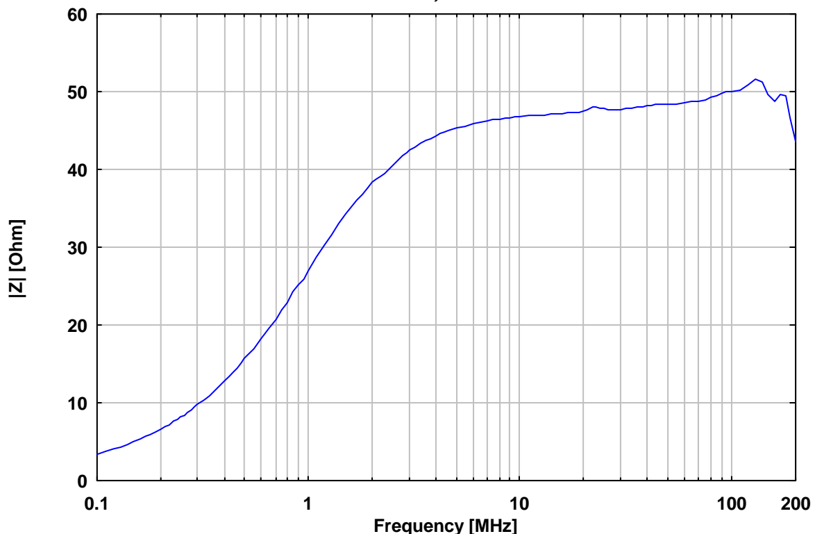
Impedanz an den Prüflingsklemmen (Kalibrieradapter KA 8125 erforderlich), BNC mit 50 Ω Abschluss, Speiseklemmen kurzgeschlossen Impedance at EuT-Terminals (Calibration Adapter KA 8125 required), BNC-Port terminated with 50 Ω, mains terminals shorted
